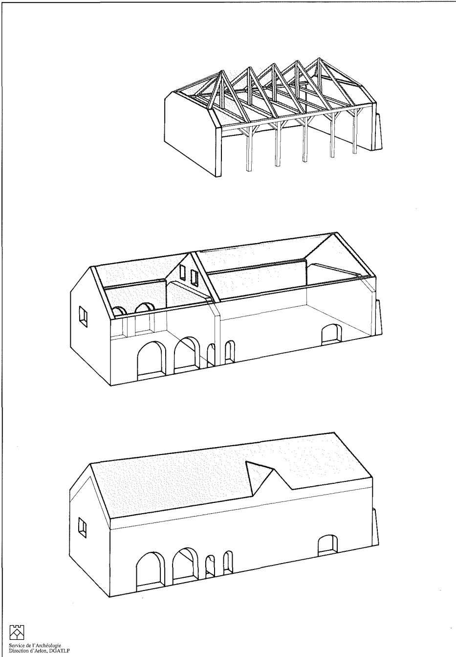
Axonométrie des trois phases de construction décelées sur le bâtiment des halles à charbon.
