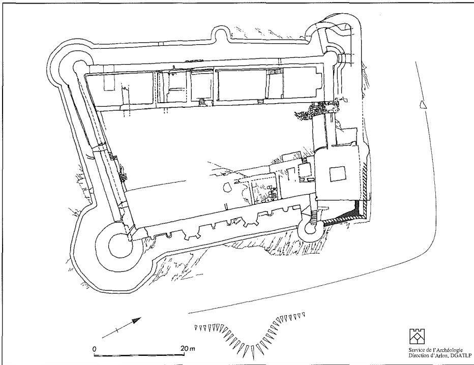
Plan général d'après A. Matthys : en noir, la courtine originelle du XIII e siècle retrouvée en fouille; en grisé, la courtine reconstruite.
